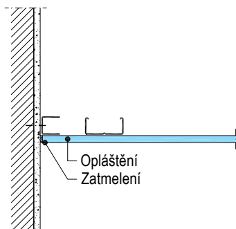
BSA 4 Napojení zavěšeného podhledu na masivní stěnu (požární odolnost zdola nebo zdola i shora).
