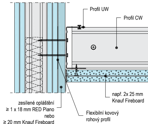
BSA 8 Napojení samonosného podhledu na lehkou příčku tl. minimálně 100 mm pro požární odolnost EI 90 a 120
