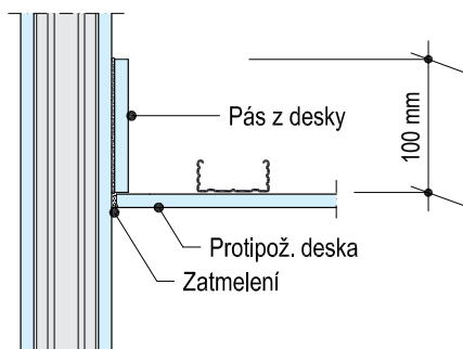
BSA 1 Napojení zavěšeného podhledu na lehké příčky (požární odolnost zdola nebo zdola i shora).
